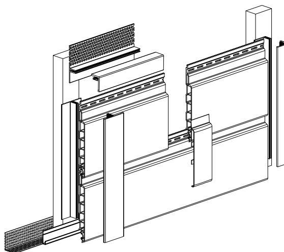
U-Profil Universal trim Épingle
