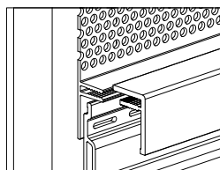
Abschlussprofil Top vent profile Profilé de finition
