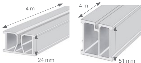
legar aluminiowy niski legar aluminiowy wysoki
