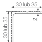
wymiary kątownika aluminiowego (mm)
