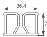
wymiary niskiego legara aluminiowego (mm)
